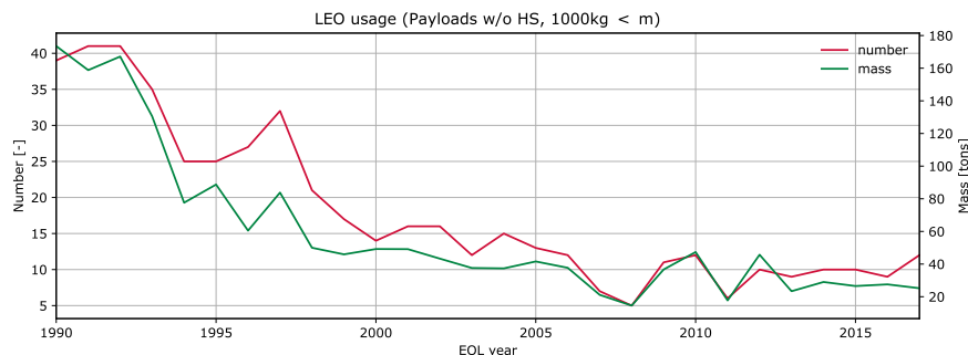
(d) Above 1000.0 kg
